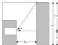
Figura 1 Valore del fattore finestra \epsilon per ostruzione frontale di fronte alla finestra di facciata
