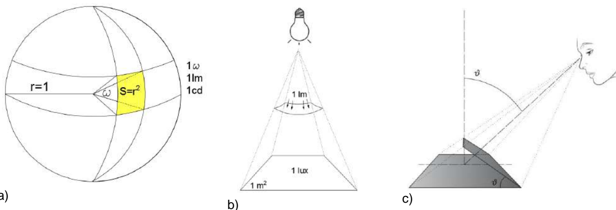
Figura 3.20: rappresentazione grafica dei parametri di intensità luminosa (a), illuminamento (b) e luminanza (c).
